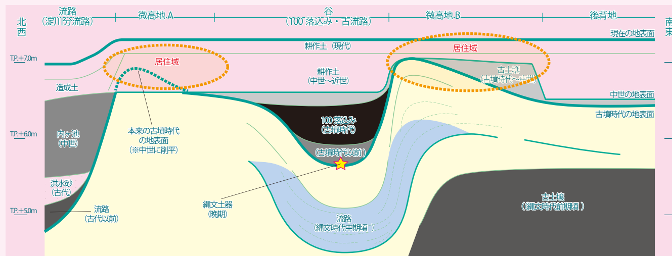
上牧遺跡における地形環境断面模式図
